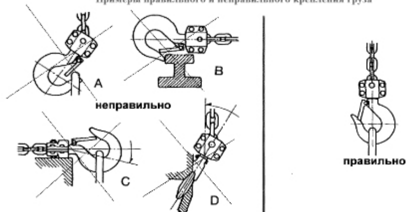
Примеры правильного и неправильного крепления груза
